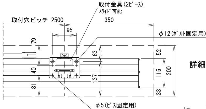
外観図 1/30
