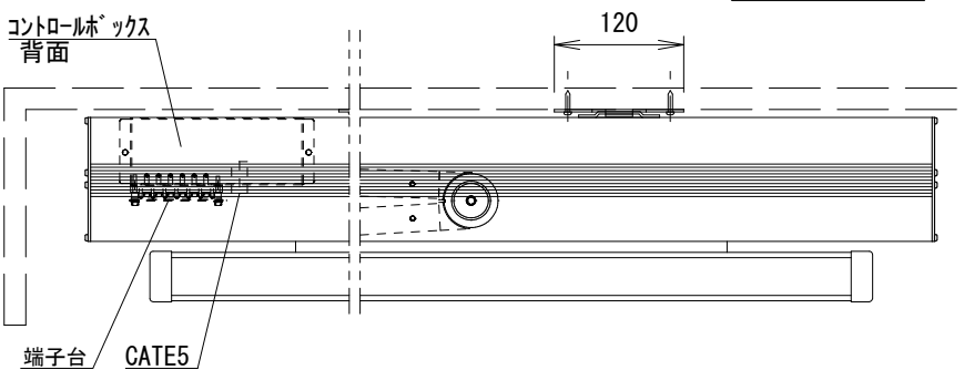
結線図
