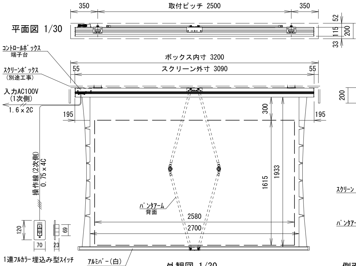
外観図 1/30
