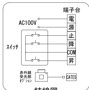
結線図
