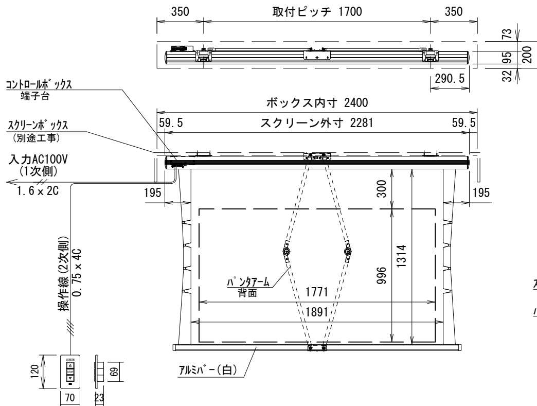
外観図 1/30
