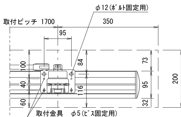
詳細図 1/8
