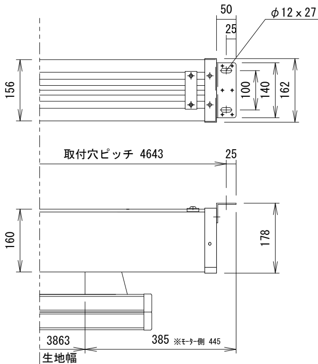
取付詳細図 1/10
