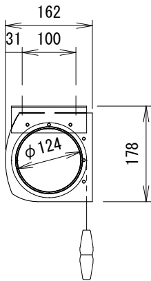
取付詳細図 1/10
