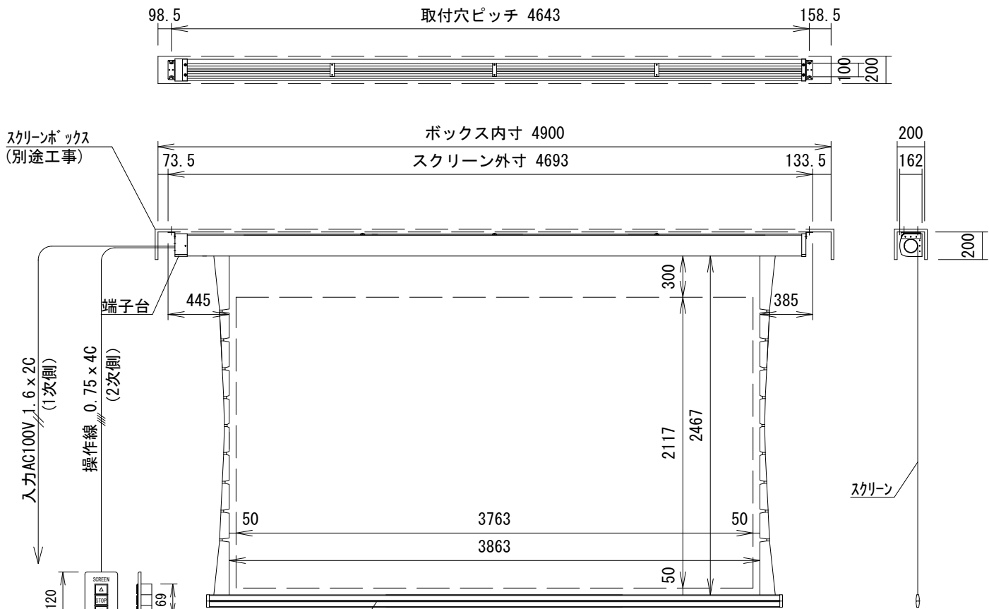
外観図 1/40
