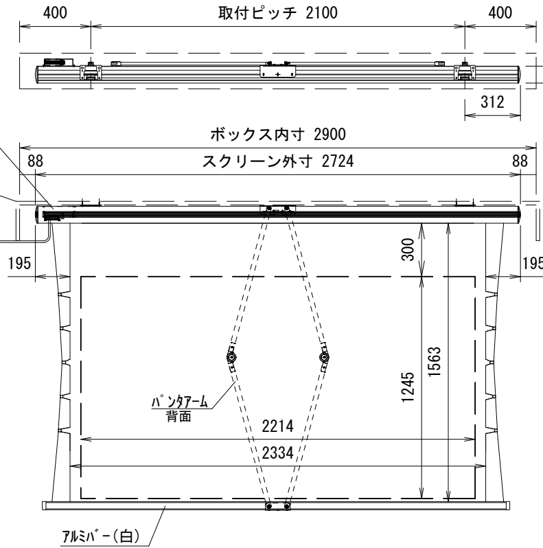
平面図 1/30
