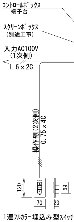
平面図 1/30
