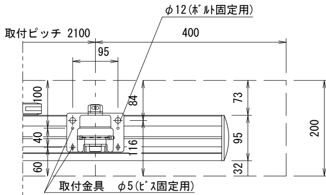
詳細図 1/8
