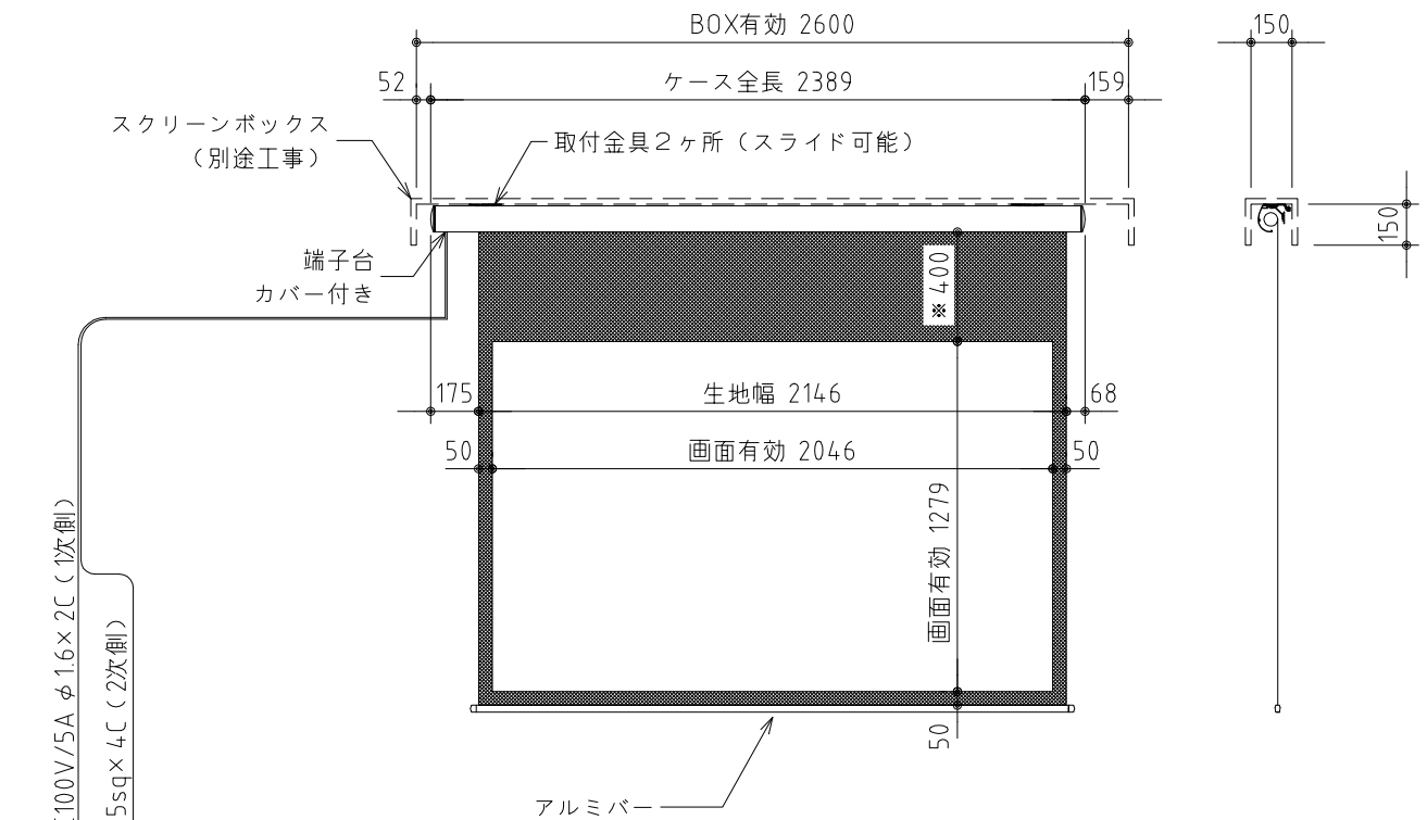
外観図 S=1/30
