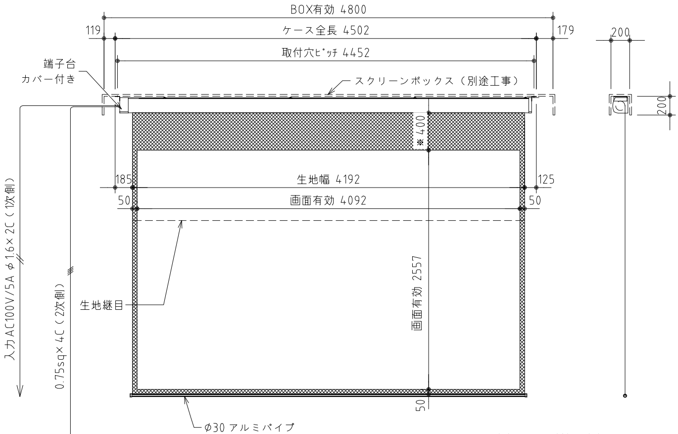
外觀図 S=1/40
