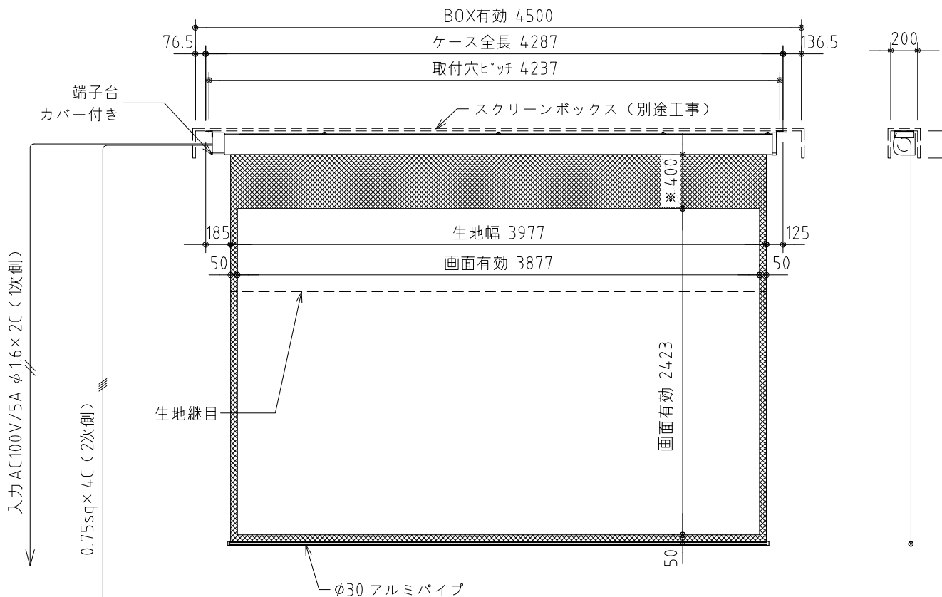
外観図 S=1/40
