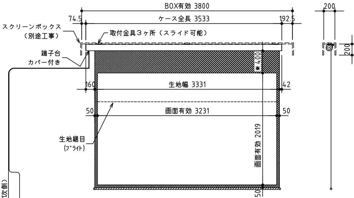
外観図 S=1/40
