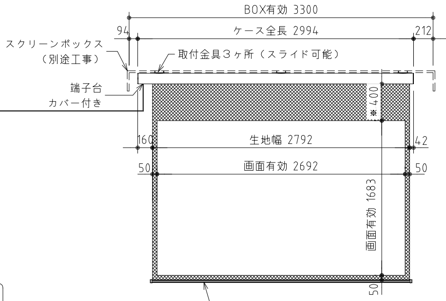
外観図 S=1/40
