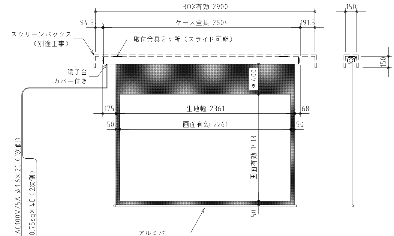
外觀図 S=1/30
