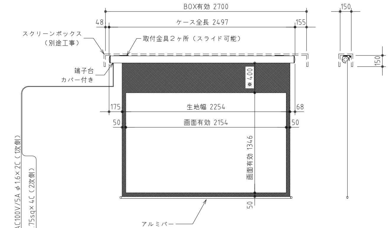
外觀図 S=1/30
