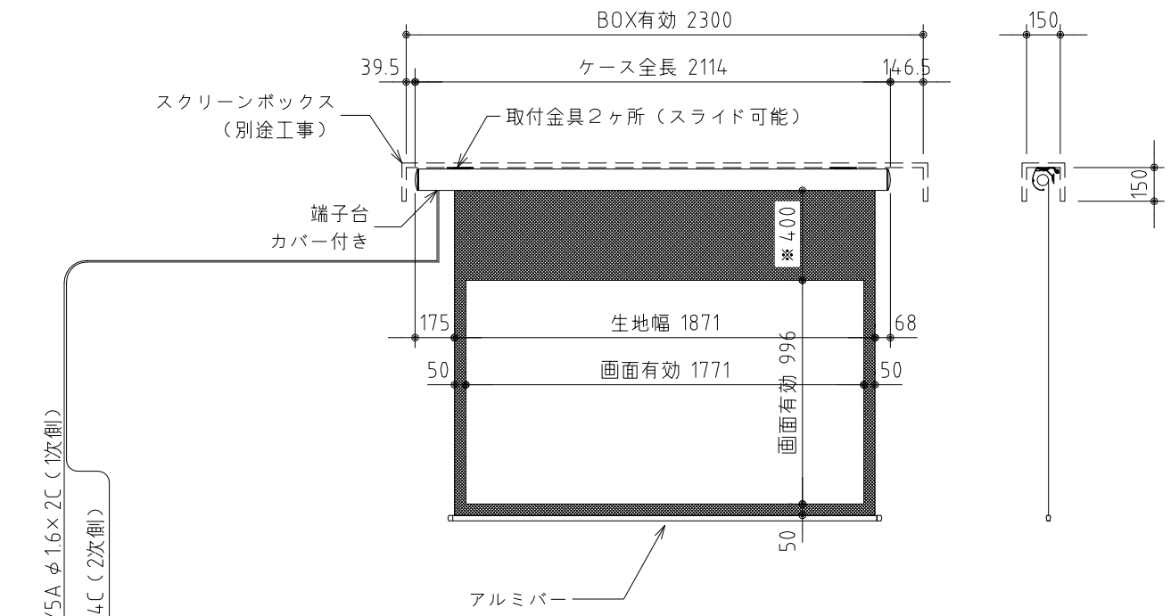
外觀図 S=1/30
