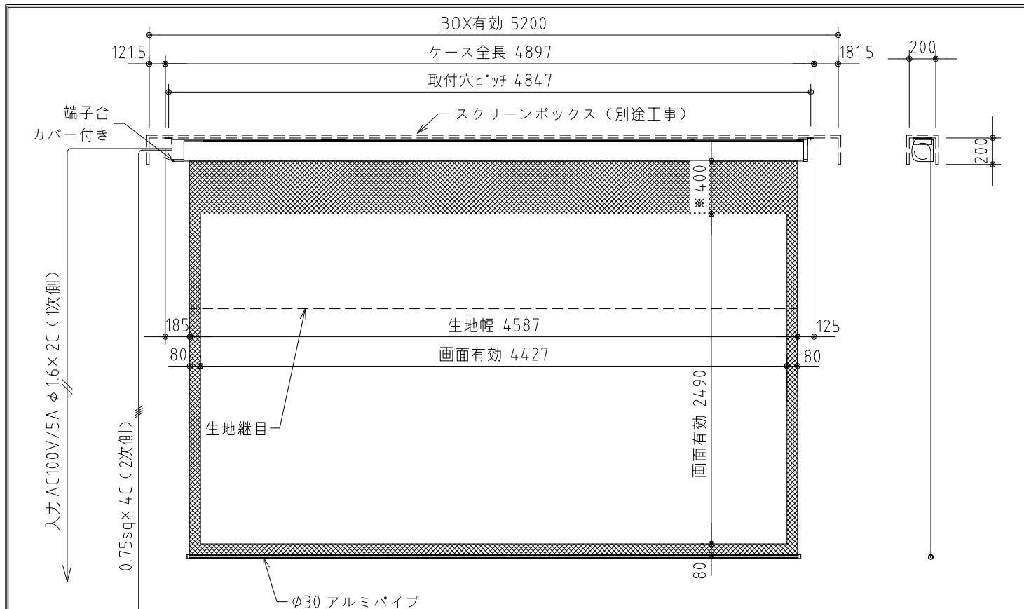
外觀図 S=1/40
