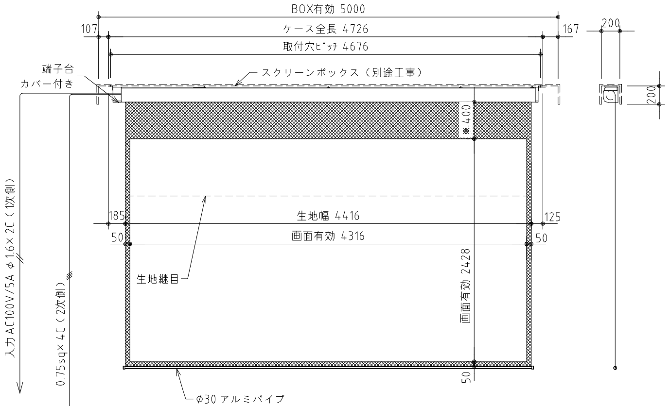
外觀図 S=1/40
