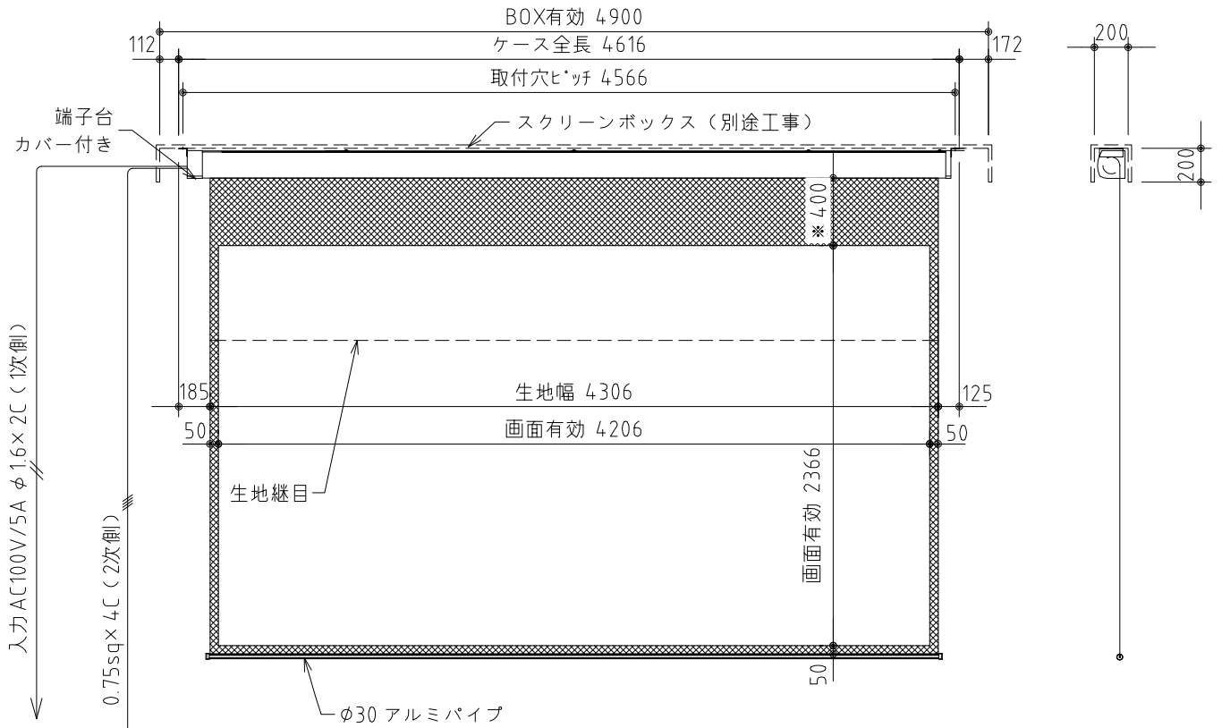
外觀図 S=1/40
