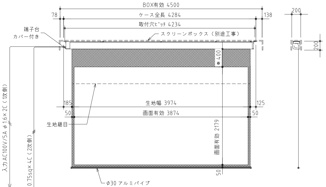
外観図 S=1/40
