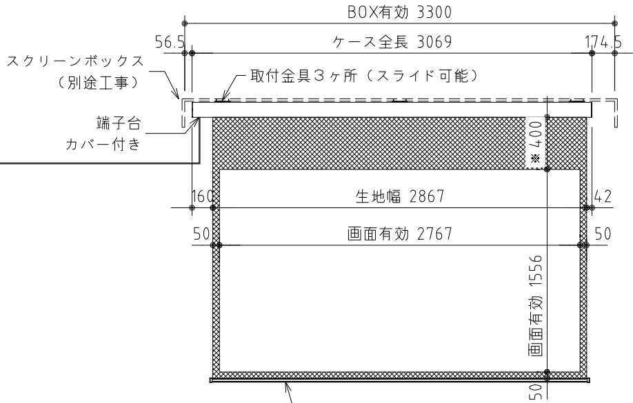
外観図 S=1/40
