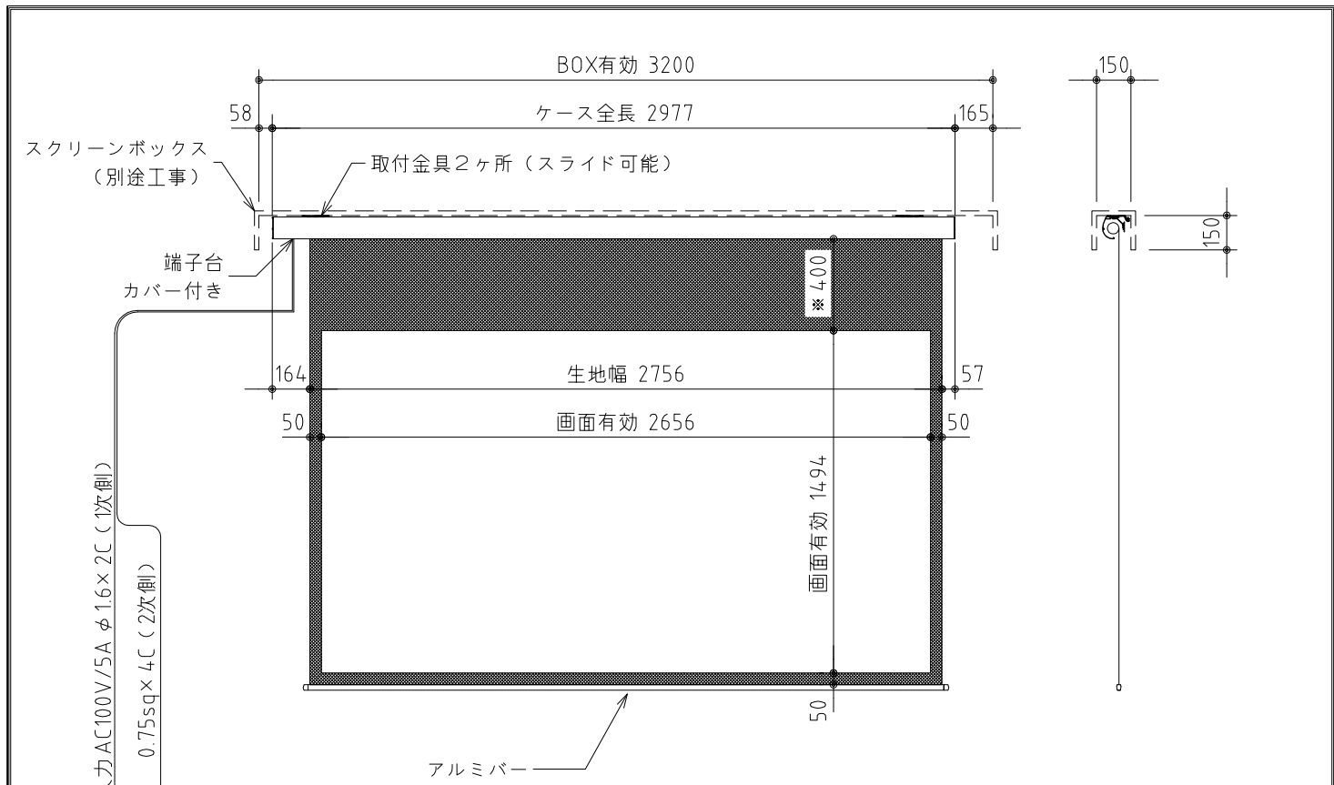
外觀図 S=1/30
