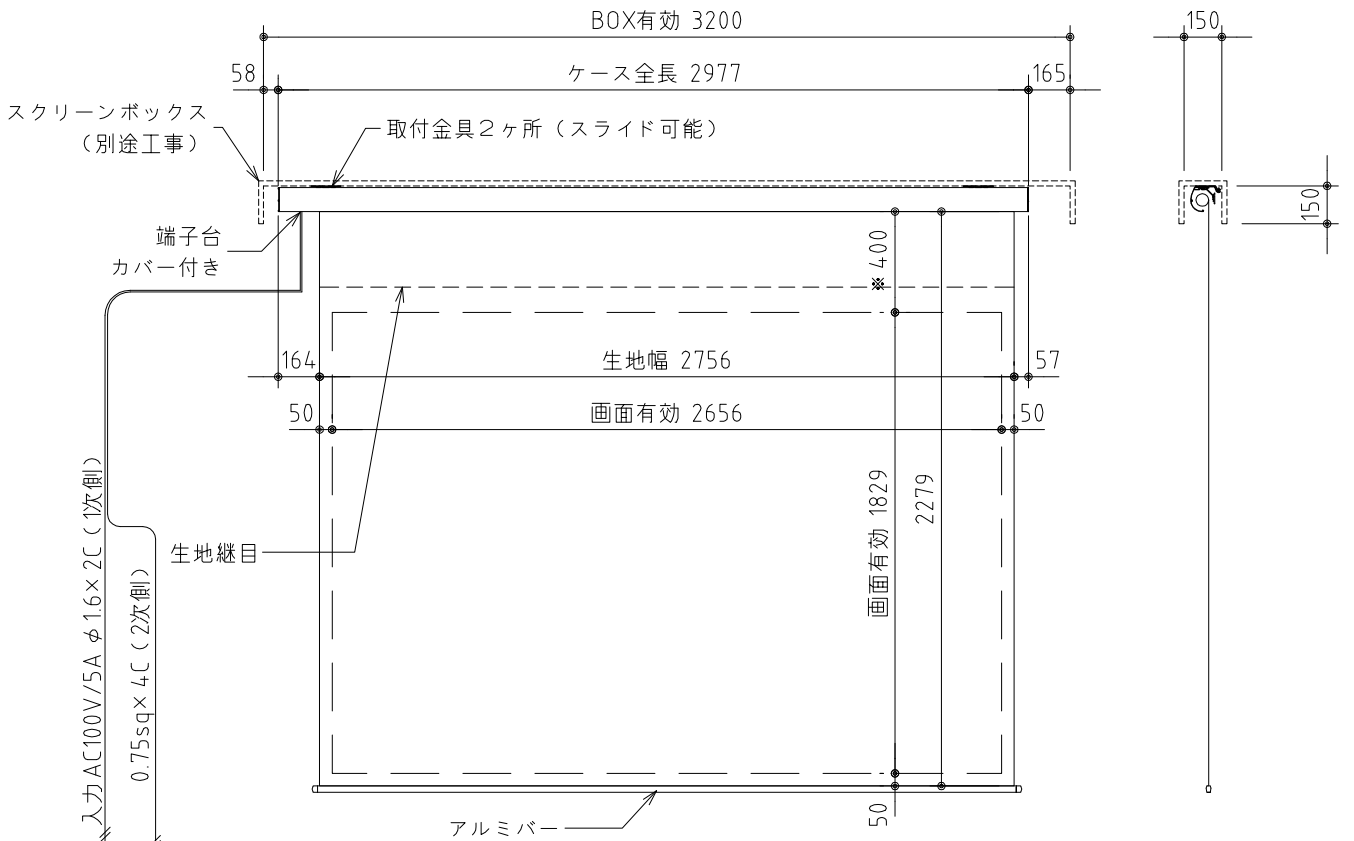
外観図 S=1/30
