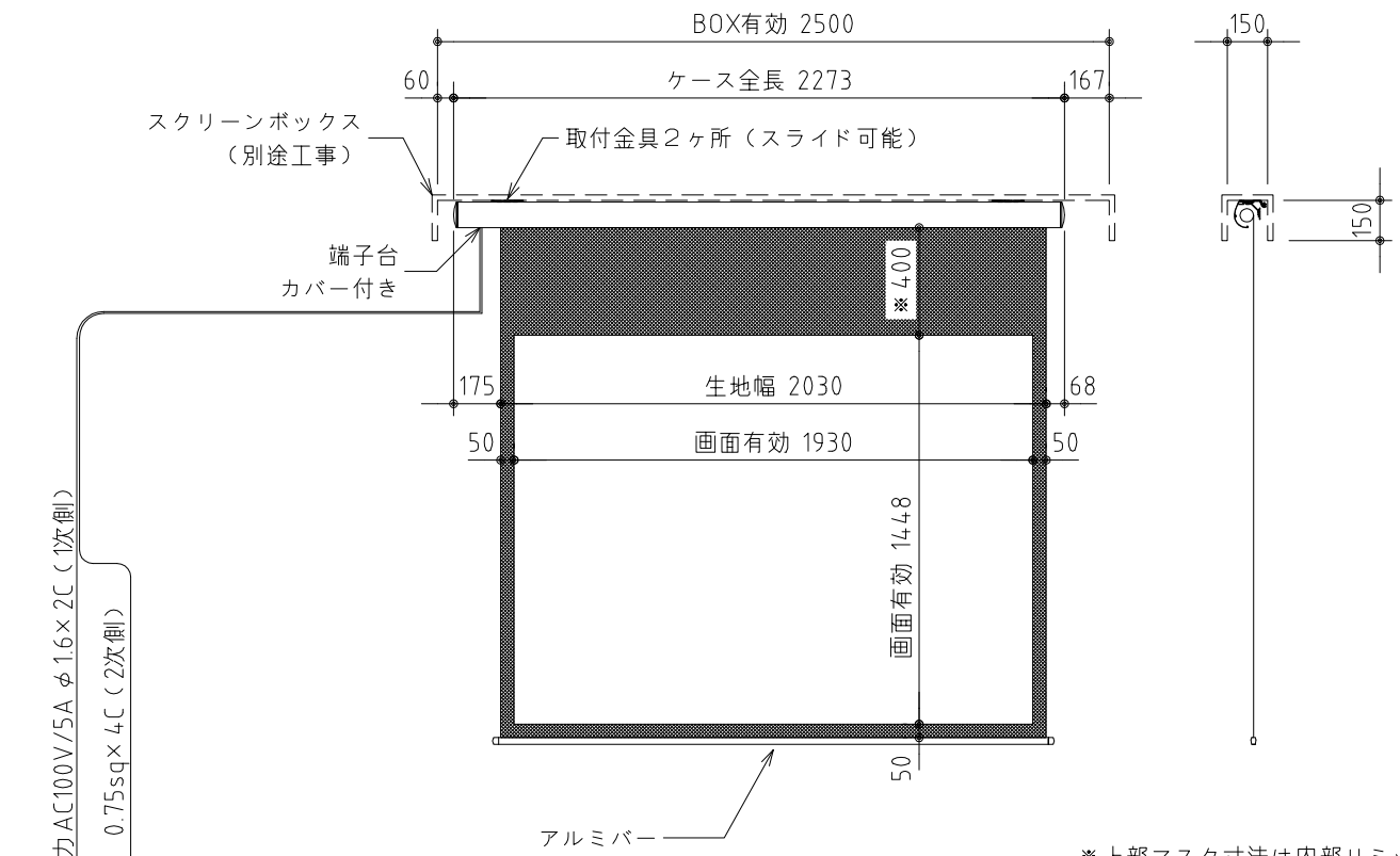
外観図 S=1/30
