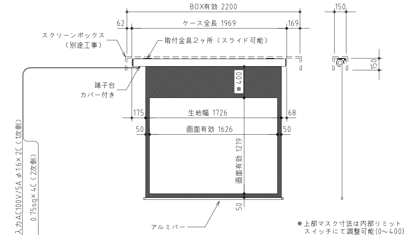
外観図 S=1/30
