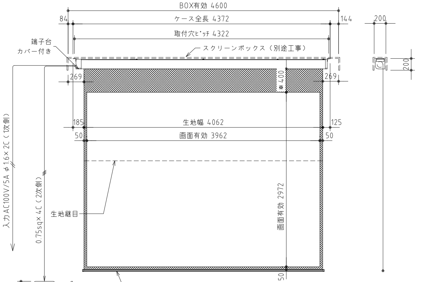
外觀図 S=1/40
