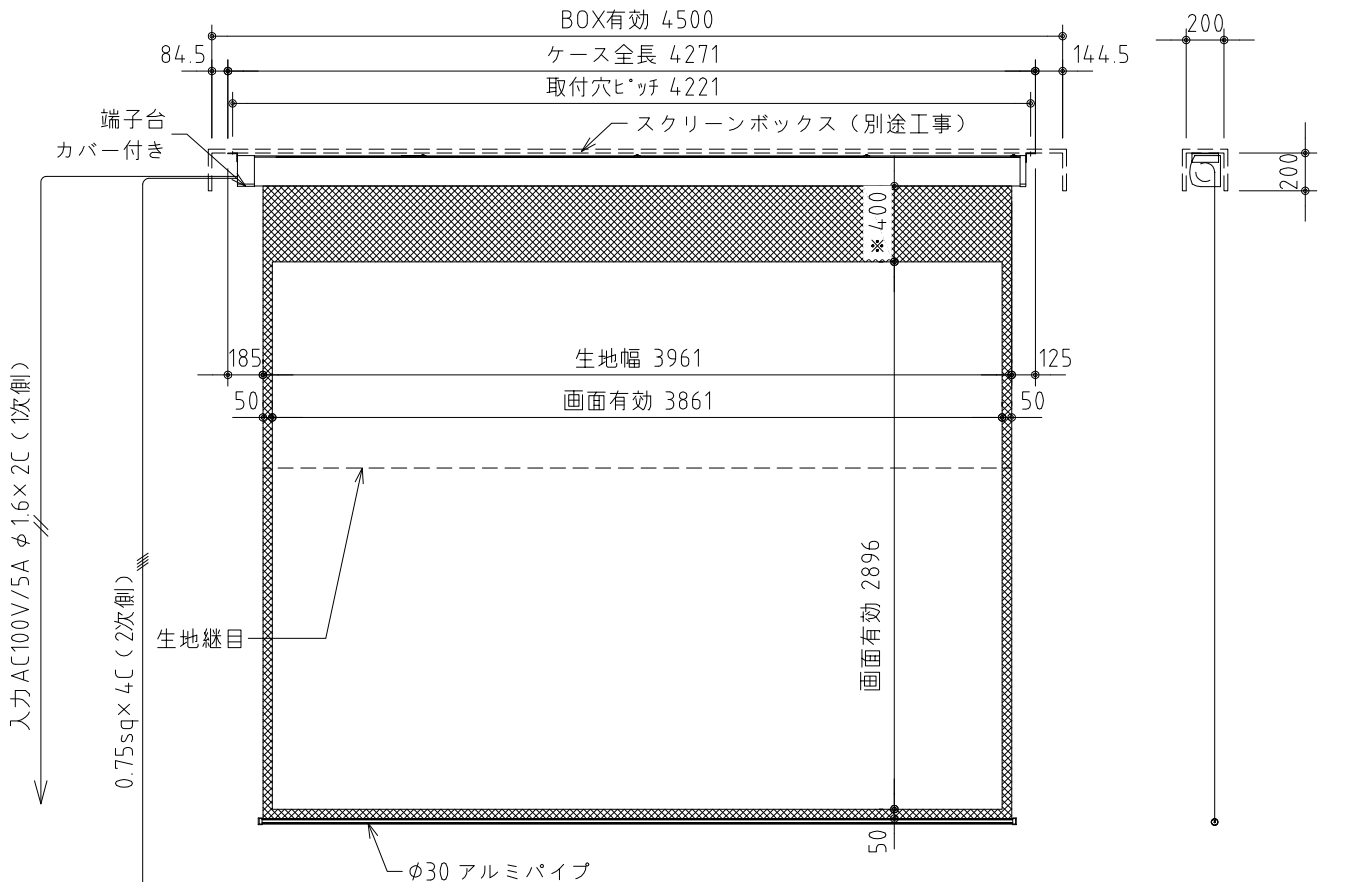
外觀図 S=1/40
