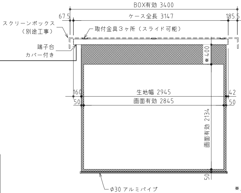
外観図 S=1/40
