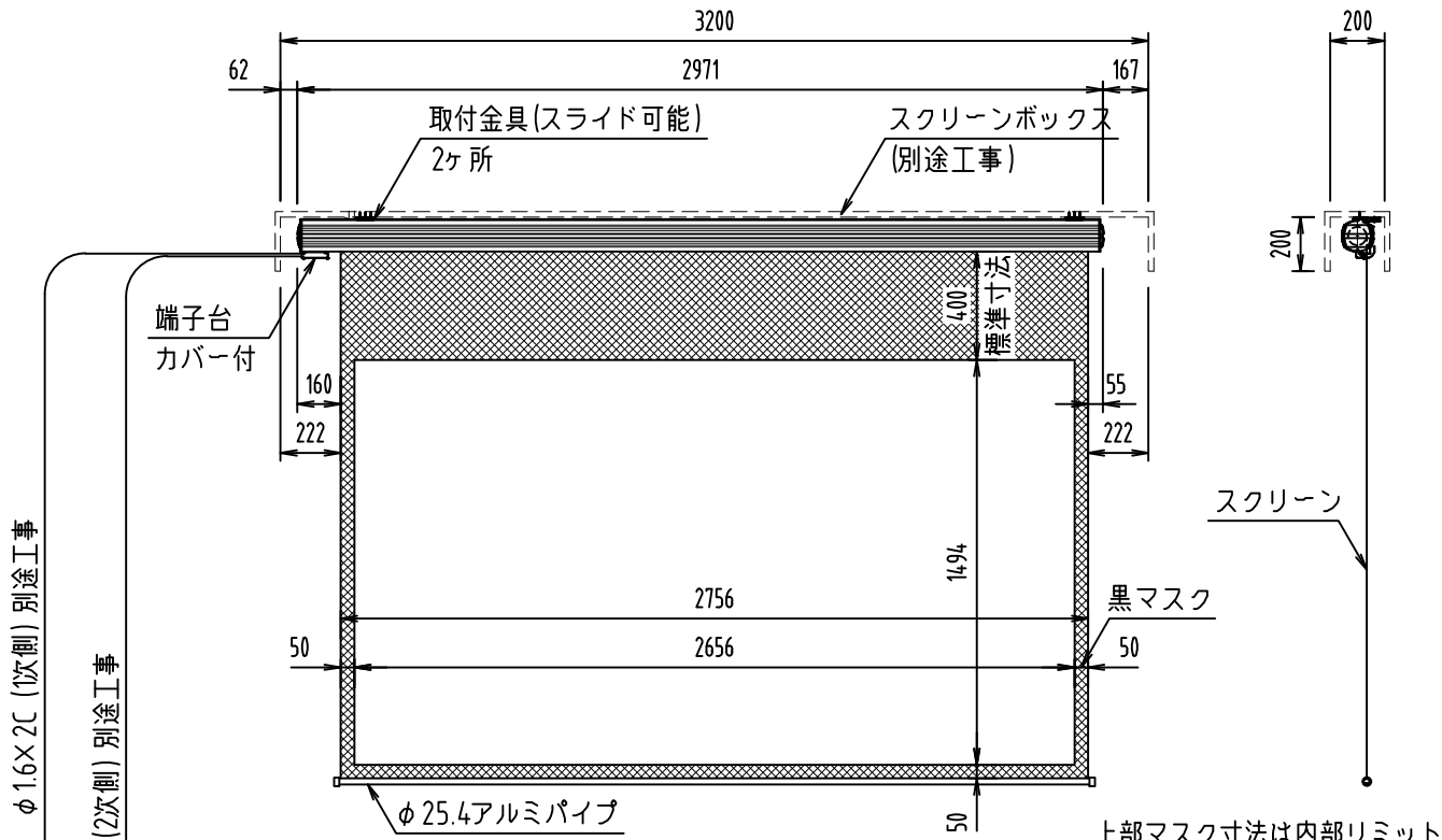
外觀図 S=1/30
