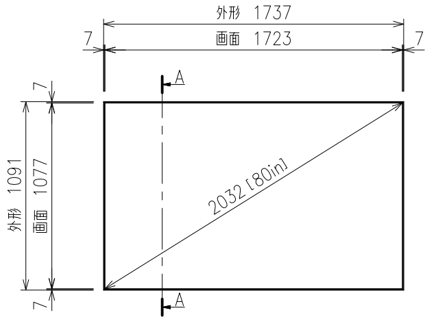
外観図（正面） S=1/30
