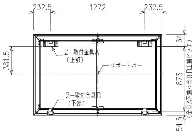
外観図（背面） S=1/30
