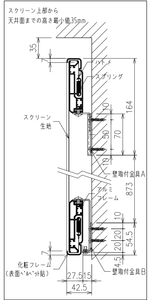
A断面詳細 S=1/4
