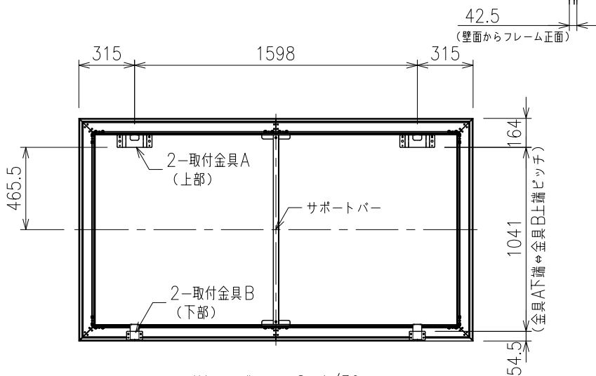
外観図(背面) S=1/30
