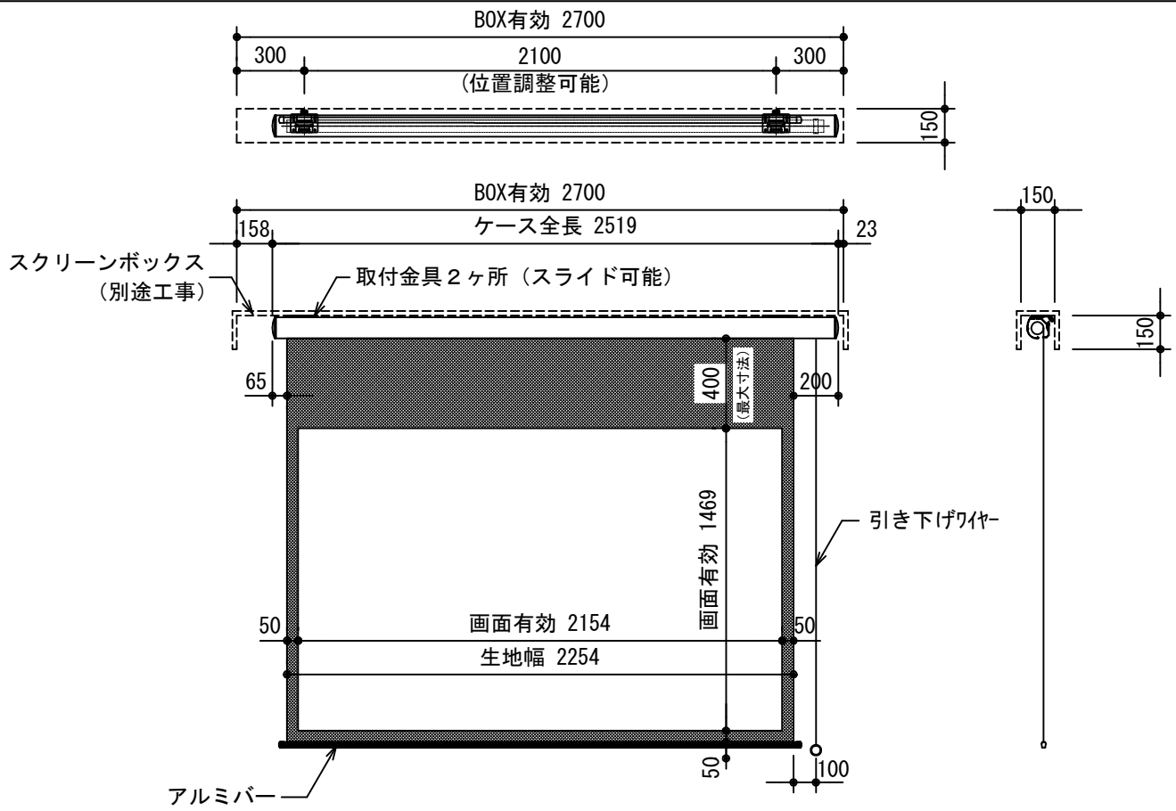
外觀図 S=1/30
