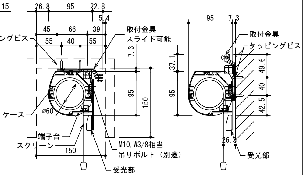
ボックス取付時 1/5
