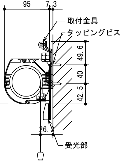
壁面取付時 1/5
