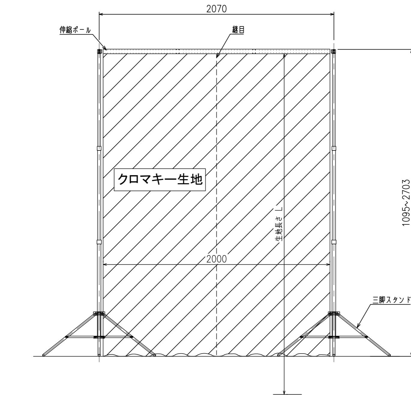
正面図
