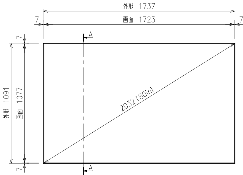
外觀図 (正面) S=1/20
