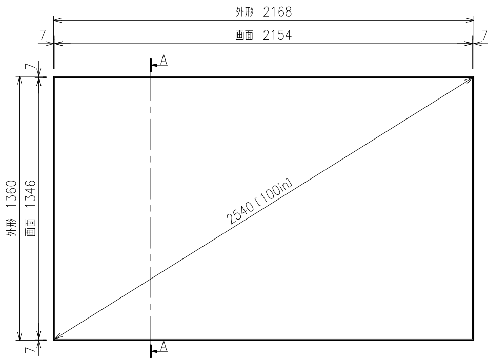
外観図 (正面) S=1/20
