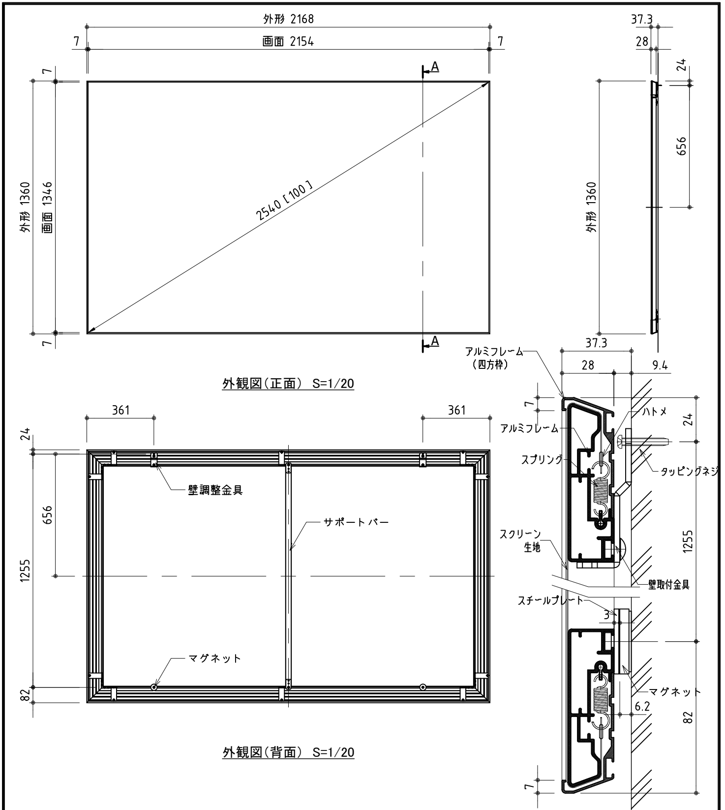
A-A断面図 S=1/2
