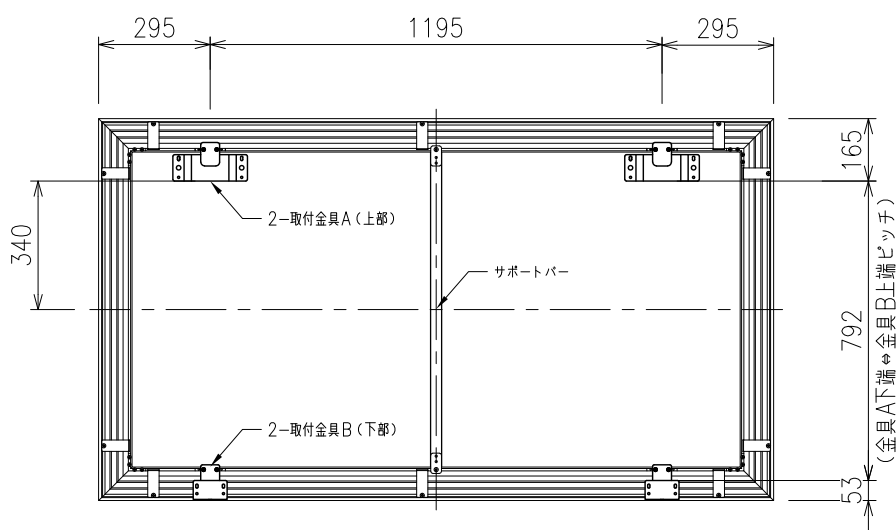
外観図(背面) S=1/20
