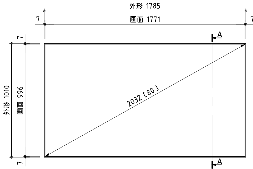
外観図(正面) S=1/20
