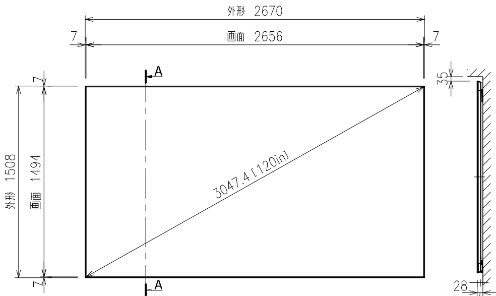
外觀図（正面） S=1/30
