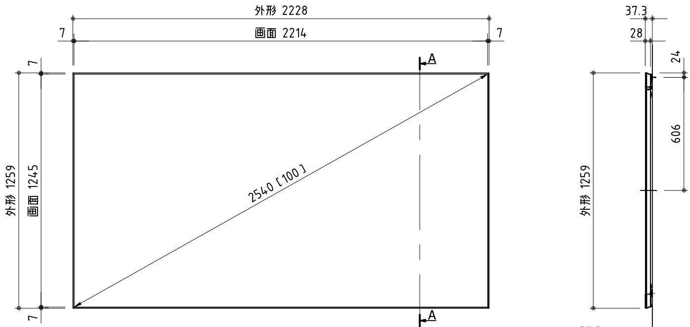
外観図(正面) S=1/20
