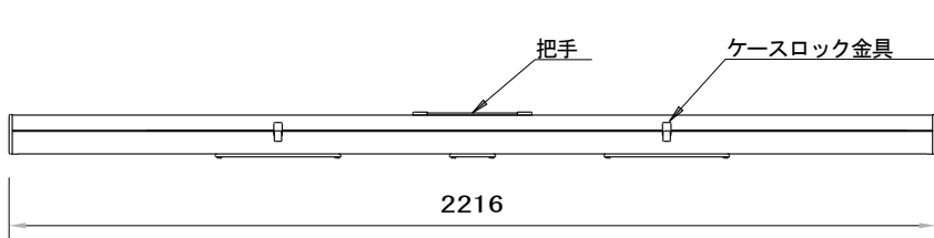
スクリーン収納時ケース外寸 S=1/20
