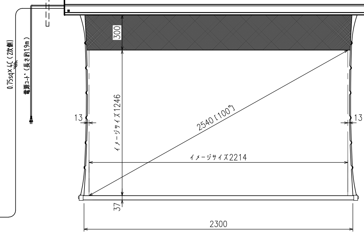
外観図 S=1/20
