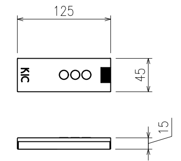
ワイヤレスリモコン S=1/5
