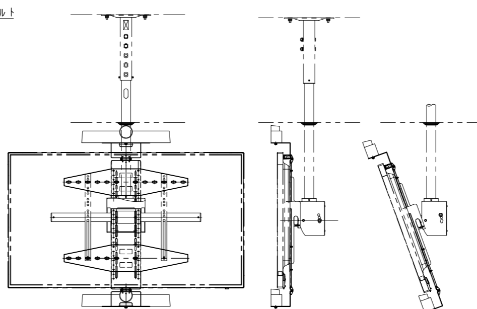
天吊設置イメージ図 S=1/20
