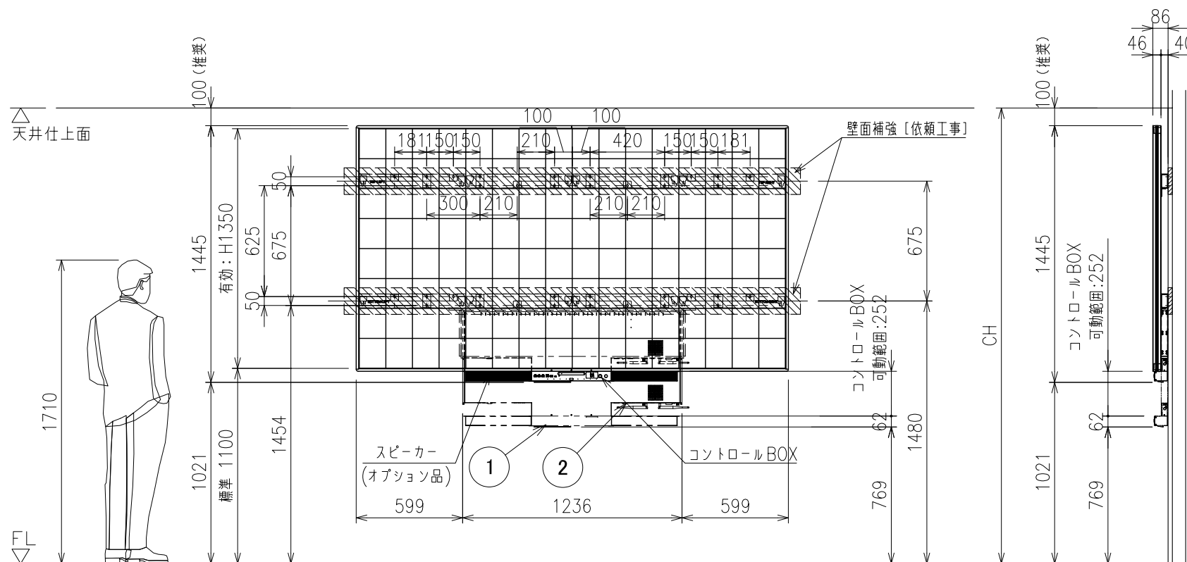
壁面設置 ※壁面意匠により壁面補強方法が異なる為、打合せが必要です。 (電源及びAVケーブル用入線開口含む)
