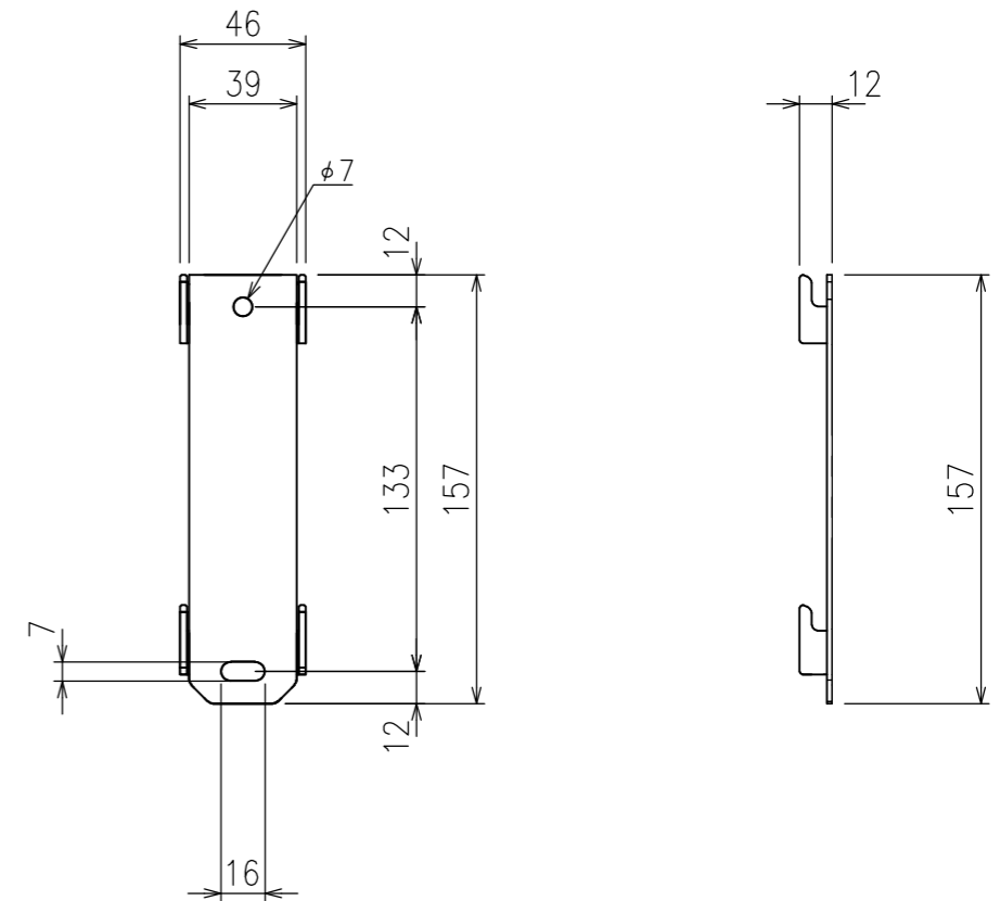
壁面取付部寸法詳細
