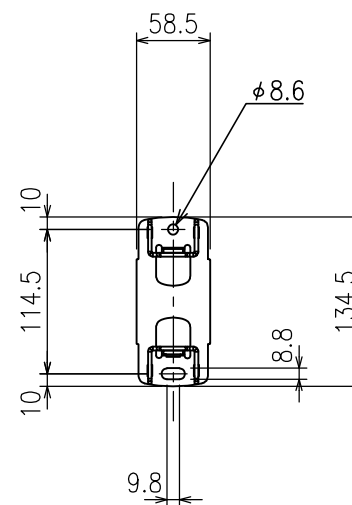
壁面取付部寸法詳細
