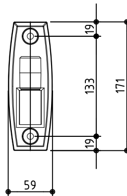
壁面取付部寸法詳細
