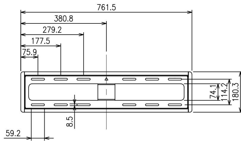
壁面取付部寸法詳細
