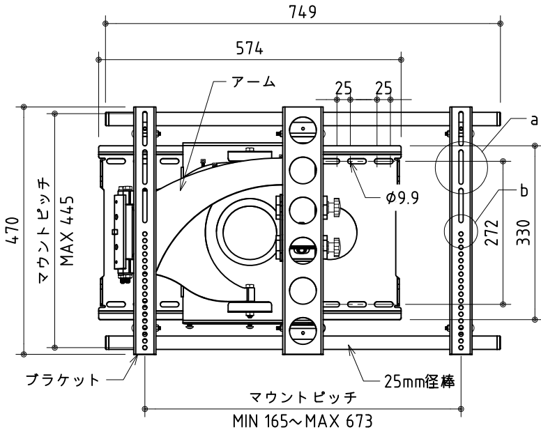
外観図 S=1/10
