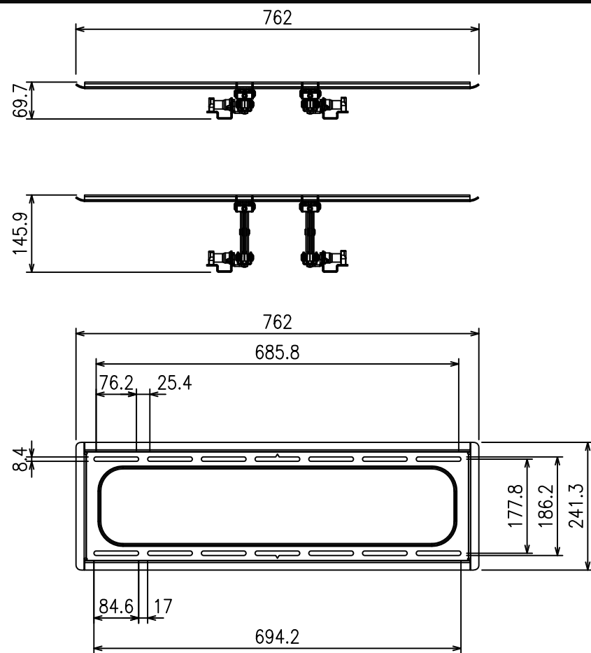
壁面取付部寸法詳細
