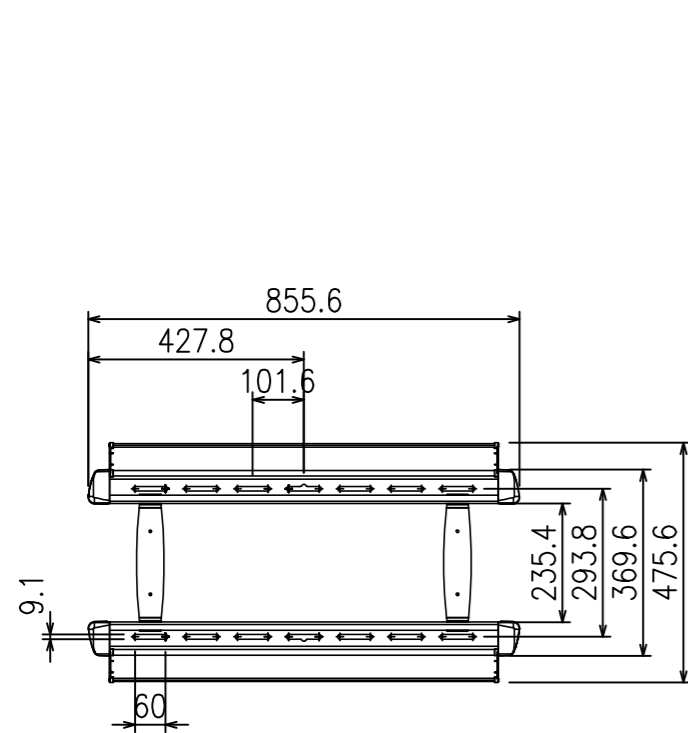
壁面取付部寸法詳細
