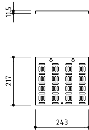
機器取付プレート図 S=1/10
