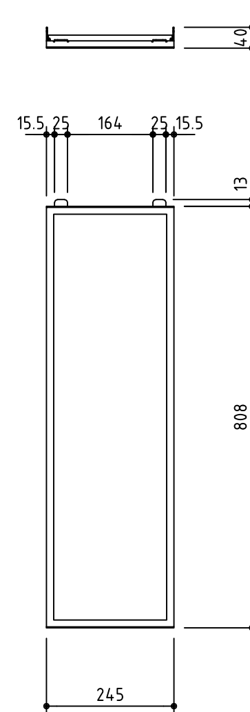
フロントパネル図 S=1/10
